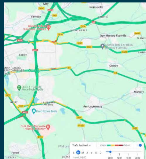
Trafic habituel en heure de pointe – Google traffic
